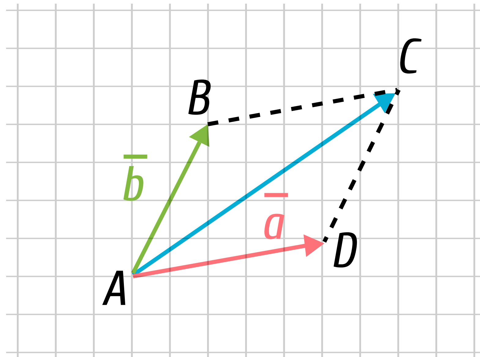
Правило паралелограма
