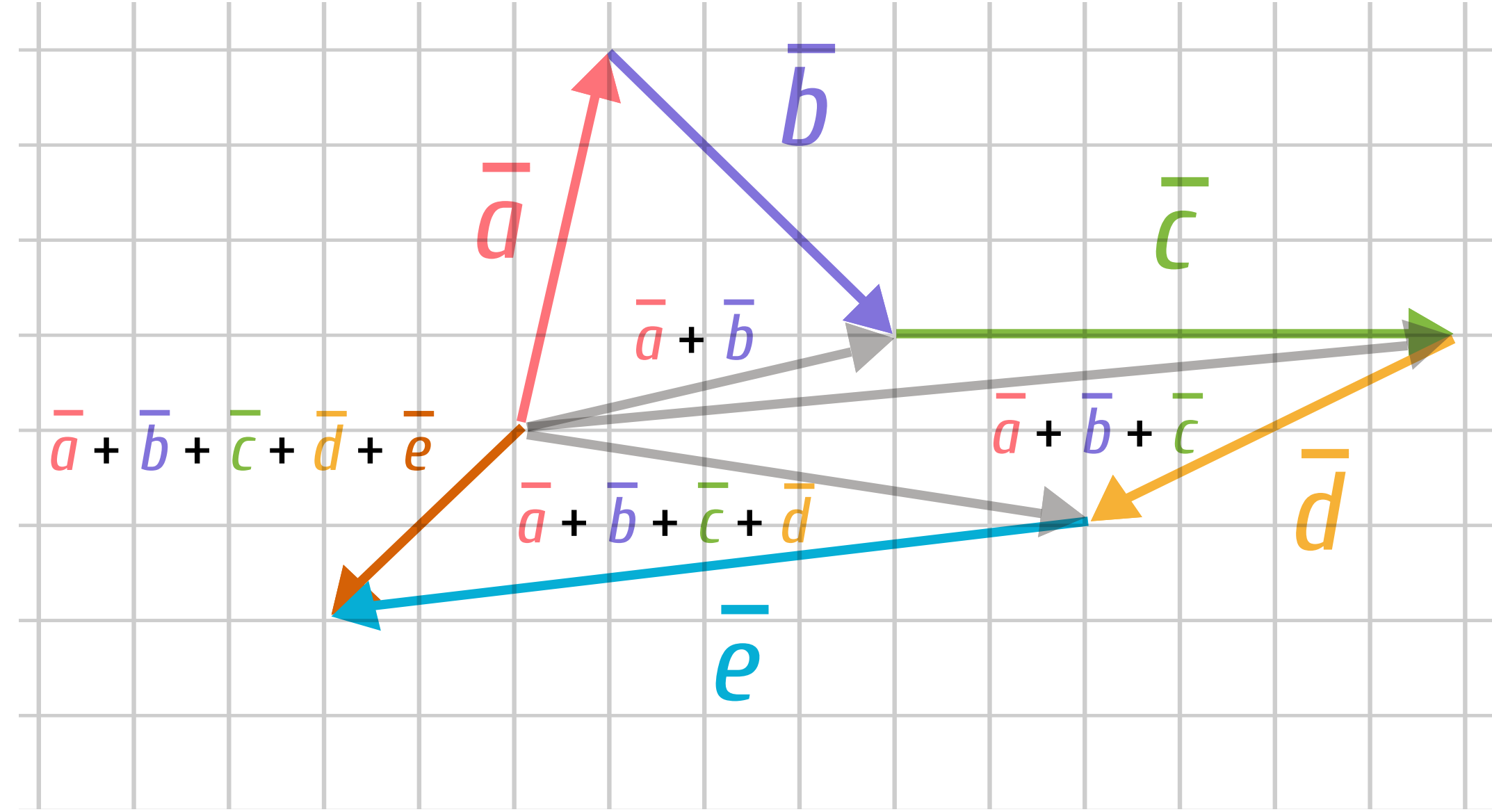
Правило многокутника
