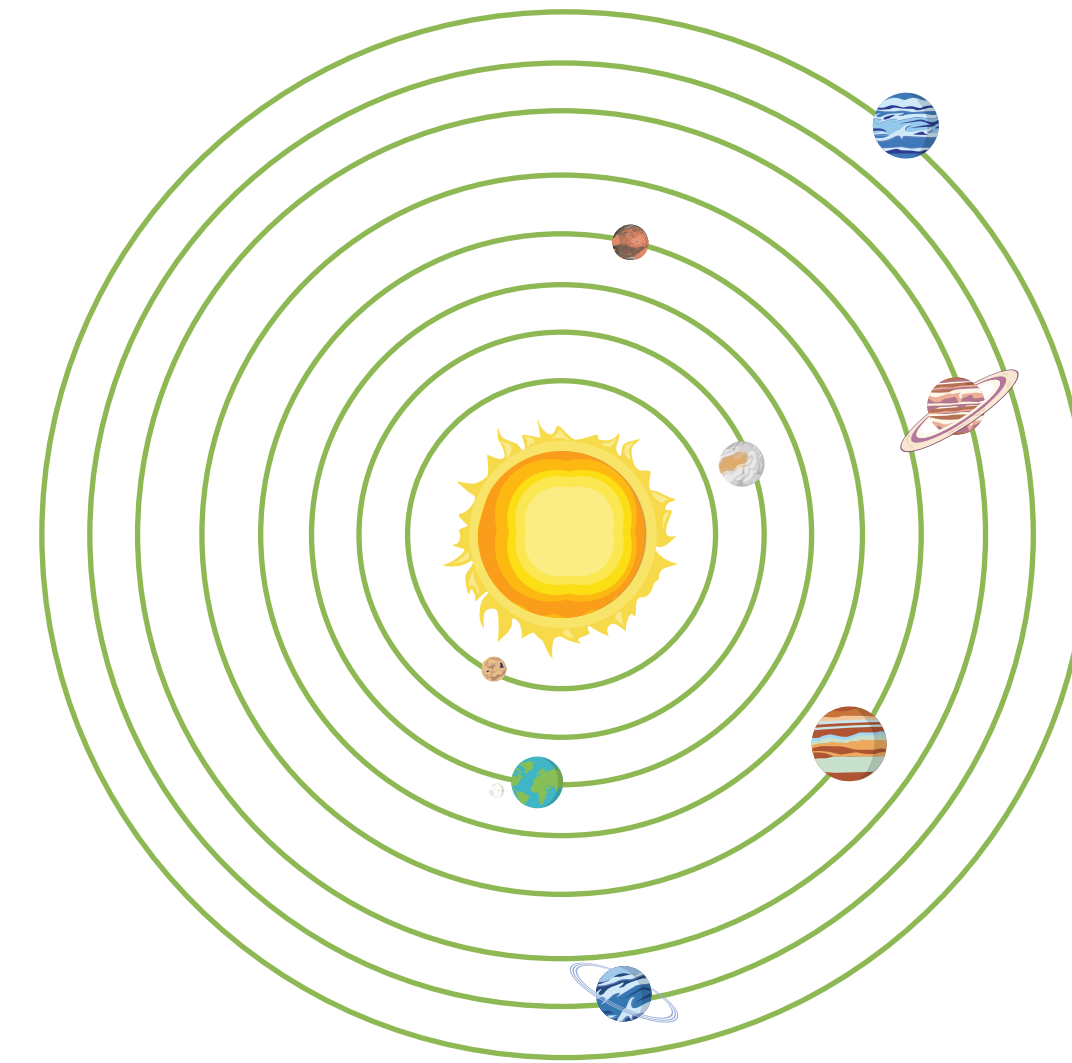
геліоцентрична система світу (Сонце в центрі Всесвіту)
