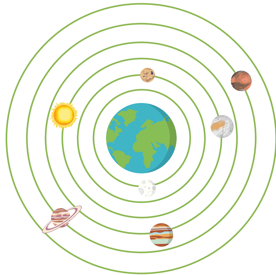
геоцентрична система світу (Земля в центрі Всесвіту)
